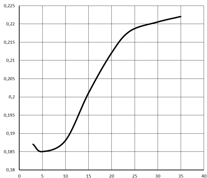
Рисунок 3.8. Зависимость излучения капли и бесконечной капельной плоскости от расстояния между ними. Упаковка капель в плоскости квадратная.
