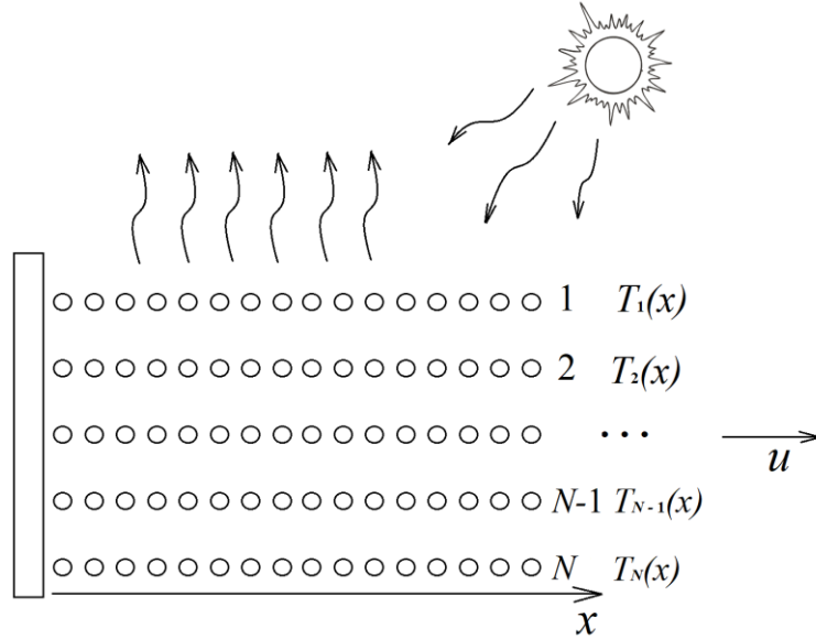
Рисунок 4.1. Остывание структурированного капельного потока, состоящего из N капельных слоёв. Температура в i – том капельном слое равна T_i(x) .
