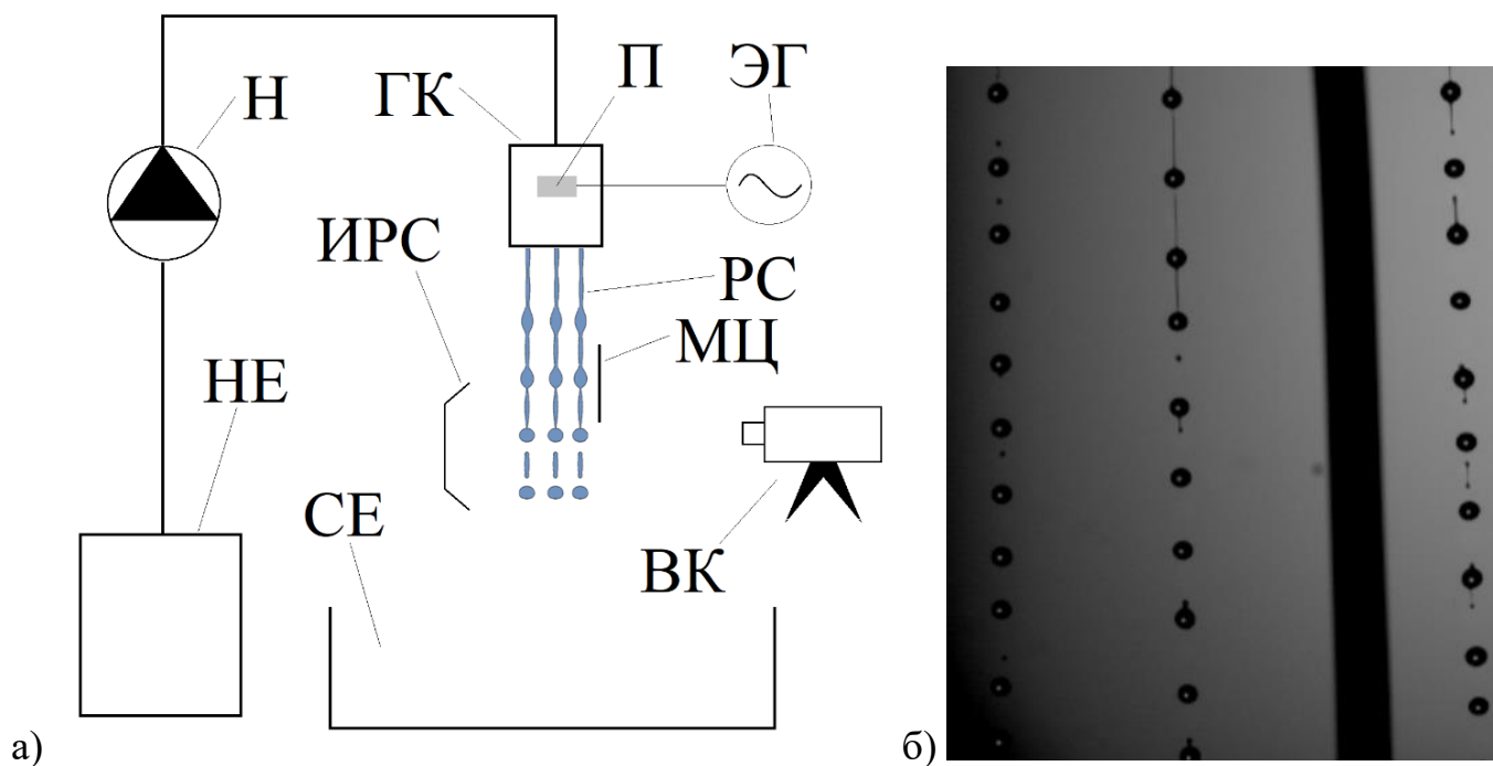
Рисунок 2.10. а) Схема экспериментальной установки. Обозначения: НЕ – термостатированная накопительная емкость, Н – перекачивающий насос, ГК – генератор капель, П – пьезоэлемент, ЭГ – генератор электрических колебаний, РС – распадающиеся на капли струи рабочего тела, СЕ – емкость для сбора рабочего тела, ИРС – источник рассеянного света, ВК – скоростная видеокамера, МЦ – мерный цилиндр. б) Фотография распадающихся на капли струй рабочей жидкости и расположенного вблизи него мерного цилиндра диаметром 1,5 мм.
