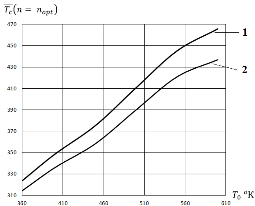
Рисунок 3.31. Зависимость конечной среднемассовой температуры капель в КХИ от их начальной температуры без учёта переоблучения элементов конфигурации (1) и с его учётом (2).
