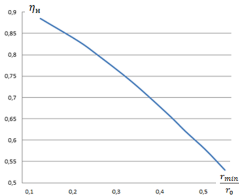
Рисунок 3.22. Численный расчет зависимости \eta_H = \eta_H(r_{min}/r_0) .
