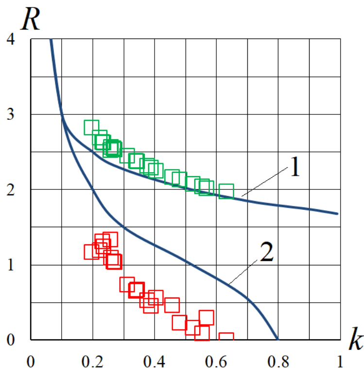
Рисунок 2.15. Линиями обозначена теоретически рассчитанная зависимость безразмерного радиуса 1 - основных и 2 - сателлитных капель от безразмерного волнового числа для не вязкого случая [77]. Зелеными и красными квадратами – экспериментально измеренная зависимость радиуса капель от безразмерного волнового числа при On = 0,6 \pm 0,15 .
