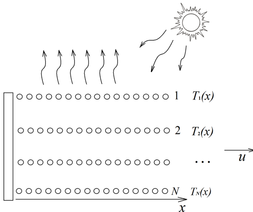
Рисунок 3.14. Остывание структурированного капельного потока.
