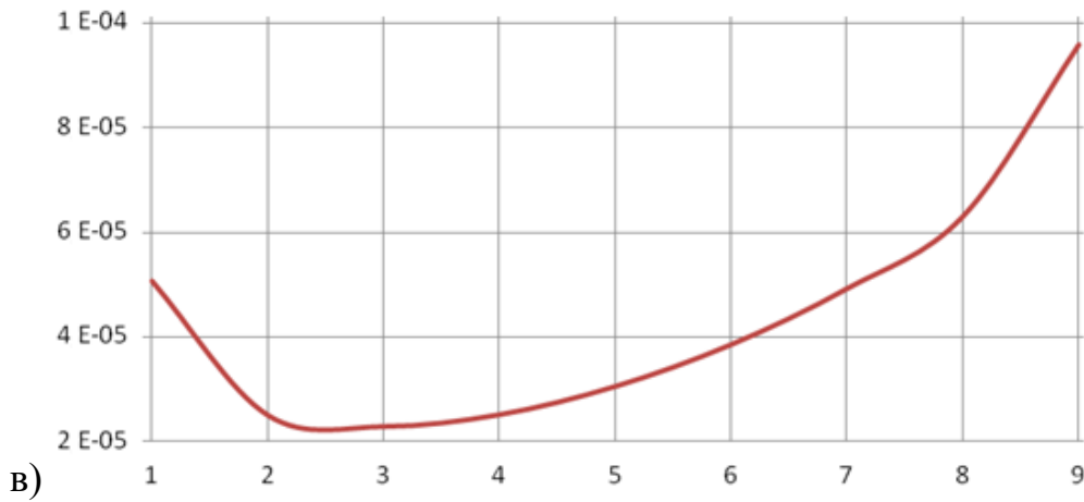
Рисунок 3.18. По оси абсцисс отложен номер капельного слоя, по оси ординат – радиус капель в метрах. Солнце светит «слева», \beta = \gamma = 4,76 . а) T_0 = 360 К, T_K = 310 К. б) T_0 = 400 К, T_K = 350 К. в) T_0 = 360 К, T_K = 310 К.
