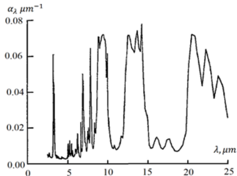
Рисунок 3.1. Зависимость коэффициента поглощения излучения \alpha_\lambda рабочего тела DC-705 при температуре 360 К [55].
