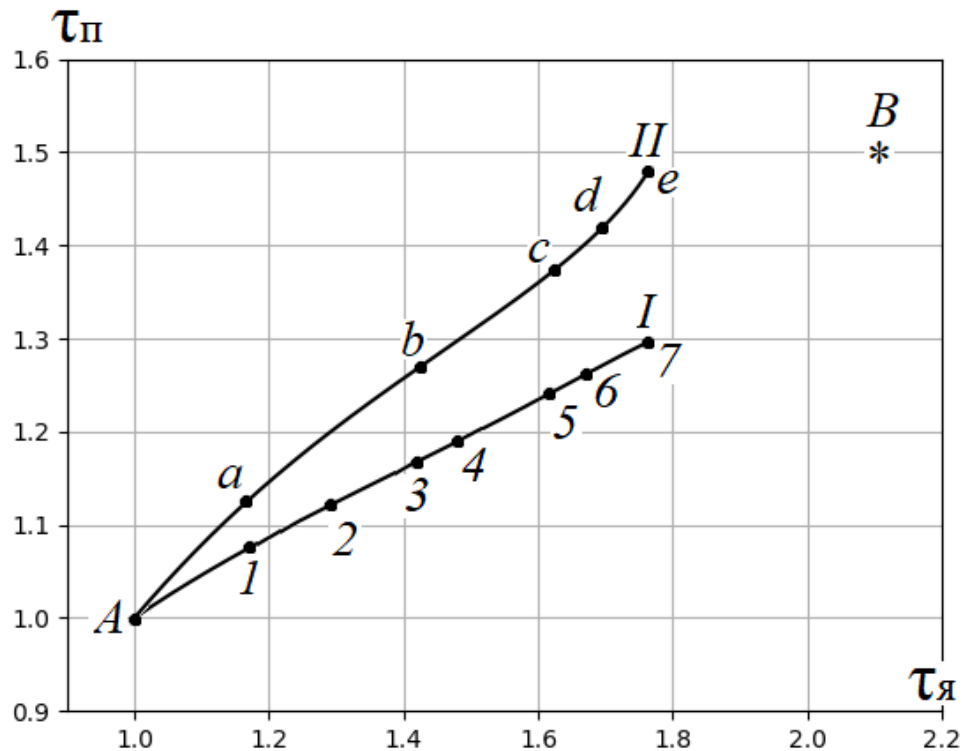
Рисунок 4.6. Результаты численного моделирования процесса установления профиля температуры: I – при отсутствии внешнего излучения, II – при наличии внешнего излучения постоянной интенсивности. A – начальная точка; конечные точки:
