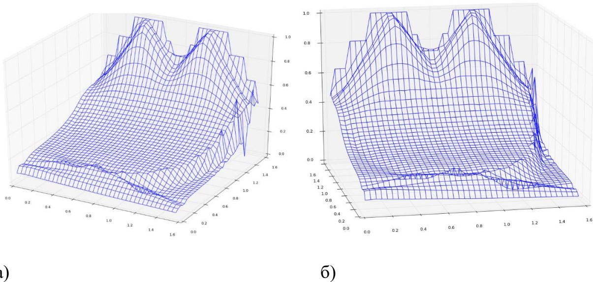
Рисунок 3.12. Элемент \psi \in [0; \pi/2] функции распределения коэффициента переоблучения капельной плоскости в двух проекциях: h = 15, \beta = \gamma = 4,76 .
