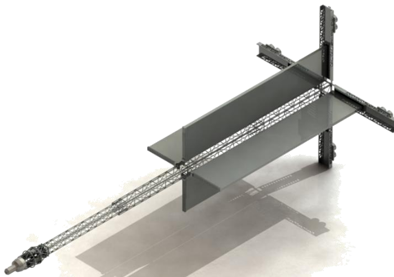
Рисунок 3.19. КХИ конфигурации «крест».
