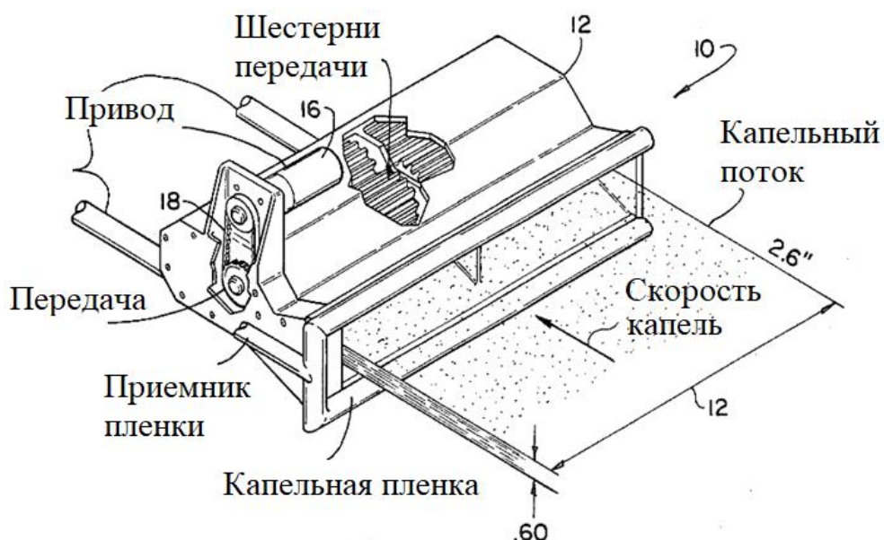
Рисунок 1.3. Пассивный уловитель капель.
