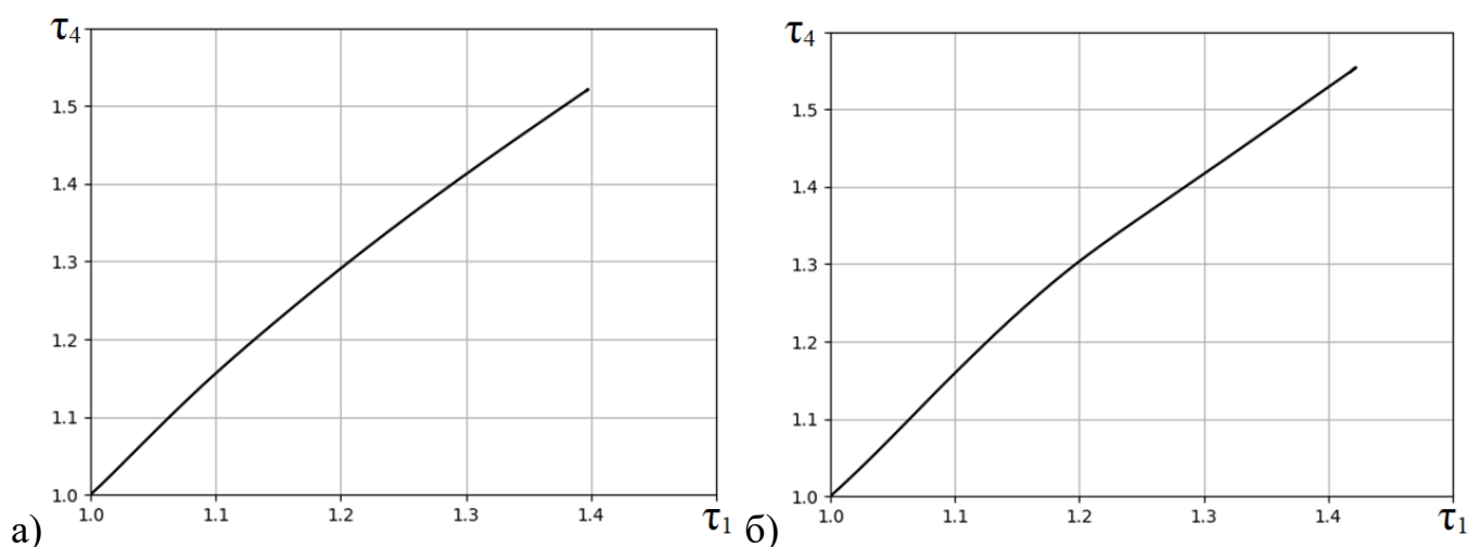
Рисунок 4.8. Траектория системы (4.4). Толщина потока: а) 0,1м и б) 0,5м.
