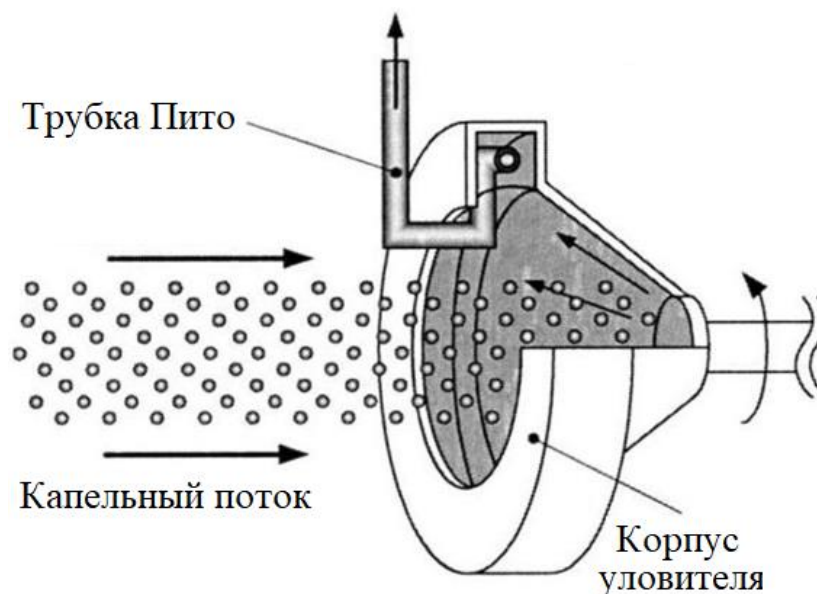
Рисунок 1.2. Центробежный уловитель капель.
