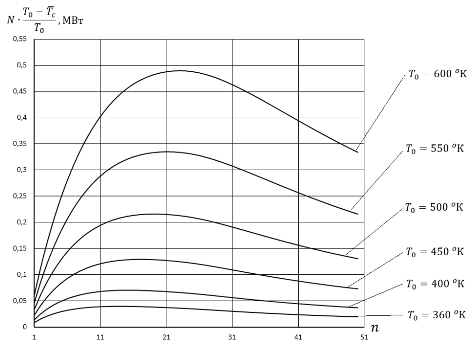
Рисунок 3.28. Зависимость \Pi = N \frac{T_0 - \bar{T}_c}{T_0} в МВт от количества капельных плоскостей n для разных начальных температур.
