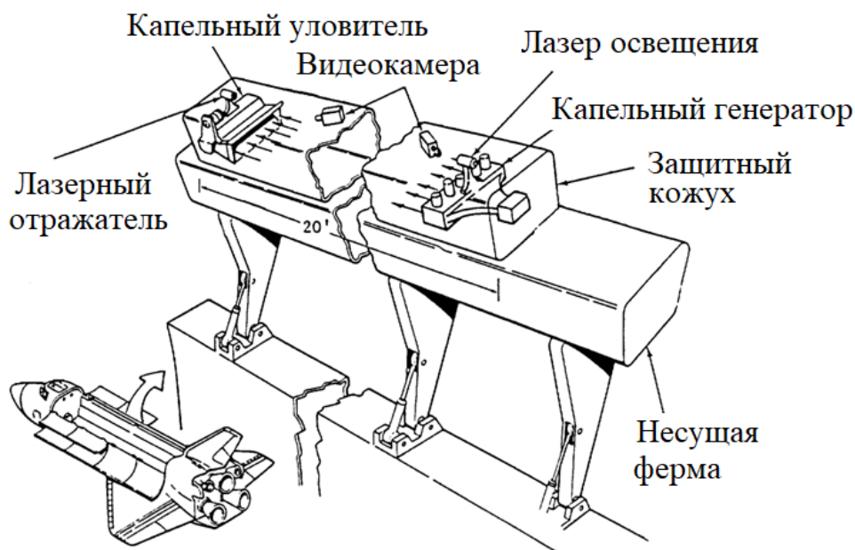
Рисунок 1.4. Схема проведения космического эксперимента с КХИ на КА «Шаттл».
