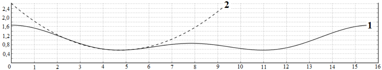
Рисунок 8. Форма распадающейся струи жидкости в момент трансформации асимптотического решения (2.38) (обозначено - 1) в автомодельное (2.56) (обозначено - 2). g = 2 , f = 0,4 , k = 0,4 .
