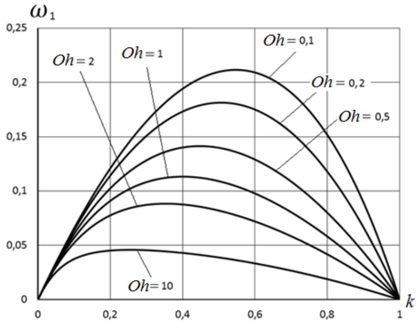
Рисунок 2.2. Зависимость фактора роста \omega_1 от безразмерного волнового числа для различных чисел Онезорге.
