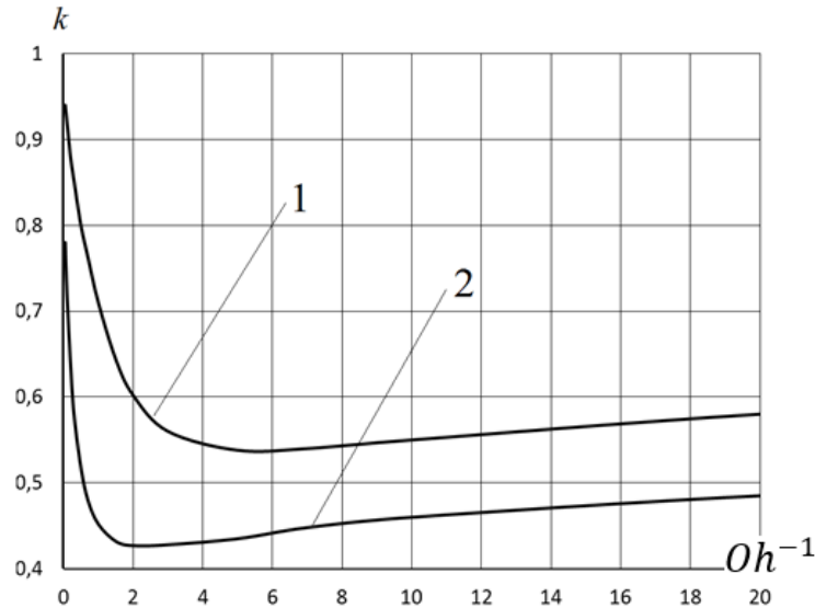
Рисунок 2.4. По оси абсцисс отложено обратное число Онезорге, по оси ординат – безразмерное волновое число. Цифрами обозначены: 1 – зависимость g(k) = 0 ; 2 – зависимость g(k) = 0,25 . Область над кривой 2 соответствует безсателлитному распаду струи.
