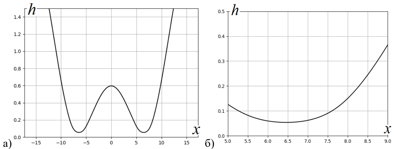
Рисунок 2.23. Форма струи в момент образования зародышей микросателлитов в разных масштабах.
