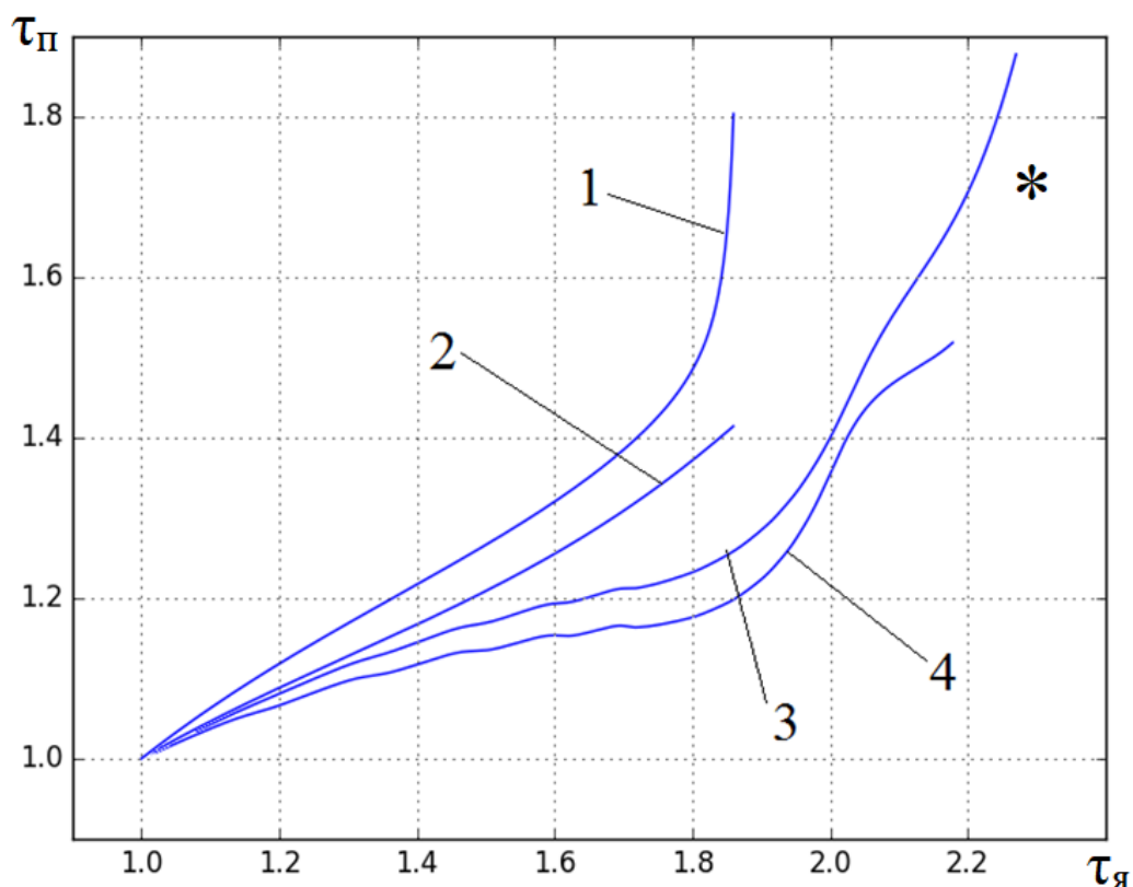
Рисунок 4.9. Численное решение системы уравнений (17). 1 – учтено солнечное излучение; 2 – без учёта солнечного излучения и дальних радиационных взаимодействий; 3 – с учетом солнечного излучения и дальних радиационных взаимодействий; 4 – учтены дальние радиационные взаимодействия; * – положение равновесия идеализированной задачи (4.10).
