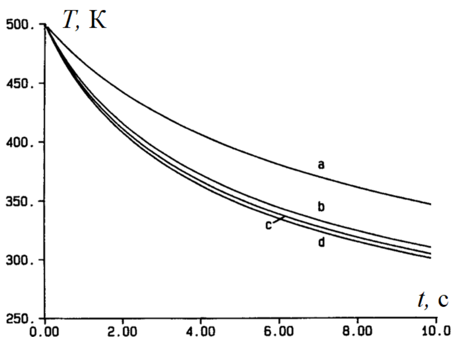
Рисунок 1.10. Зависимость среднемассовой температуры капельных потоков от времени. Рабочее тело – масло DC-705, диаметр капель – 100 мкм. Оптическая толщина потоков: а) \tau = 1 ; б) \tau = 0,1 ; в) \tau = 0,01 ; д) одиночная капля [55].
