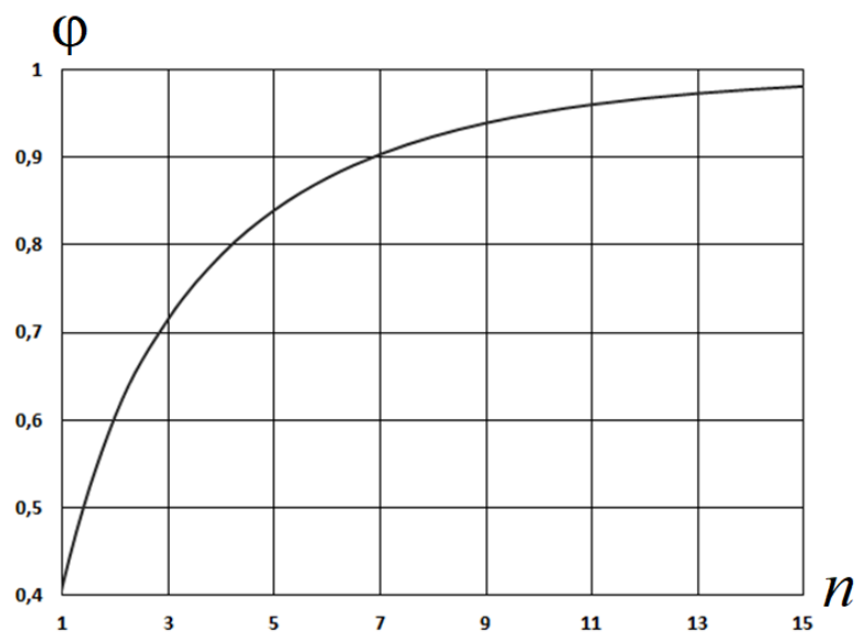
Рисунок 3.21. Зависимость коэффициента поглощения излучения набора капельных плоскостей \varphi от их количества n ; \beta = \gamma = 4,76 , \varepsilon = 1 .
