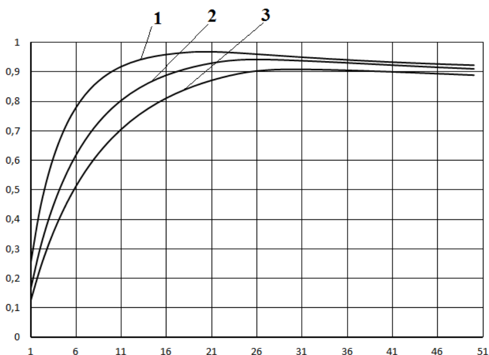
Рисунок 3.35. Зависимость излучательной способности капельного потока от числа капельных плоскостей для структур с различным расстоянием между капельными струйками. Начальная температура капель равна 360 К. Расстояние между капельными струйками \gamma : 1- 4,76; 2- 7,5; 3 - 10,0.
