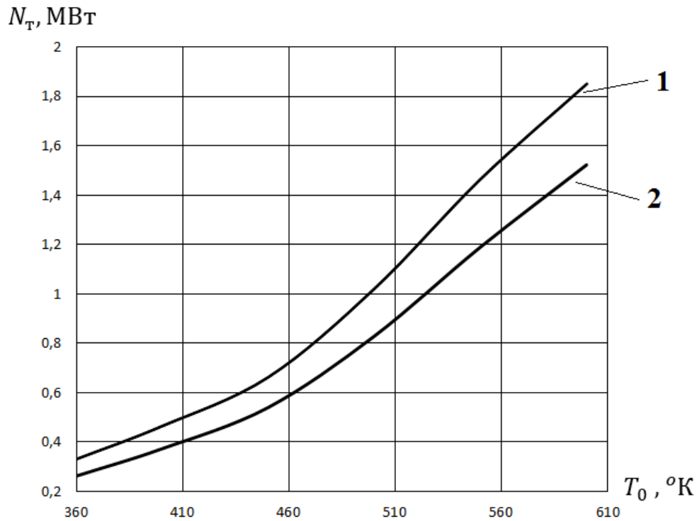
Рисунок 3.30. Зависимость мощности КХИ без учёта переоблучения элементов конфигурации (1) и с его учётом (2).
