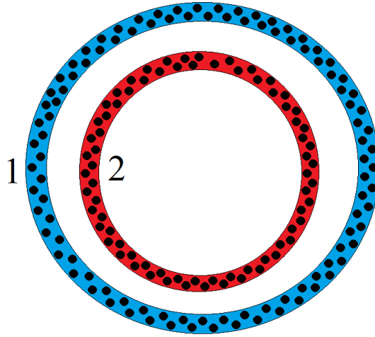
Рисунок 4.3. Модель капельного потока, состоящего из периферии (1) и ядра (2).
