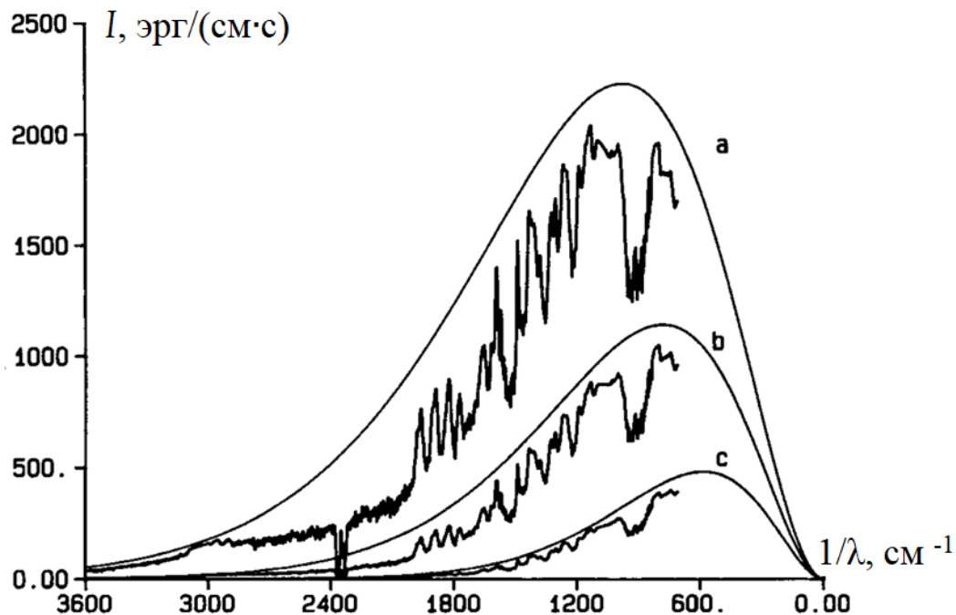
Рисунок 1.9. Спектральная интенсивность поглощения излучения капель DC-705 диаметром 100 мкм при разных температурах [55]. Температура капли: а) 500 К; б) 400 К; в) 300 К. Гладкие линии- интенсивность излучения абсолютно чёрного тела.
