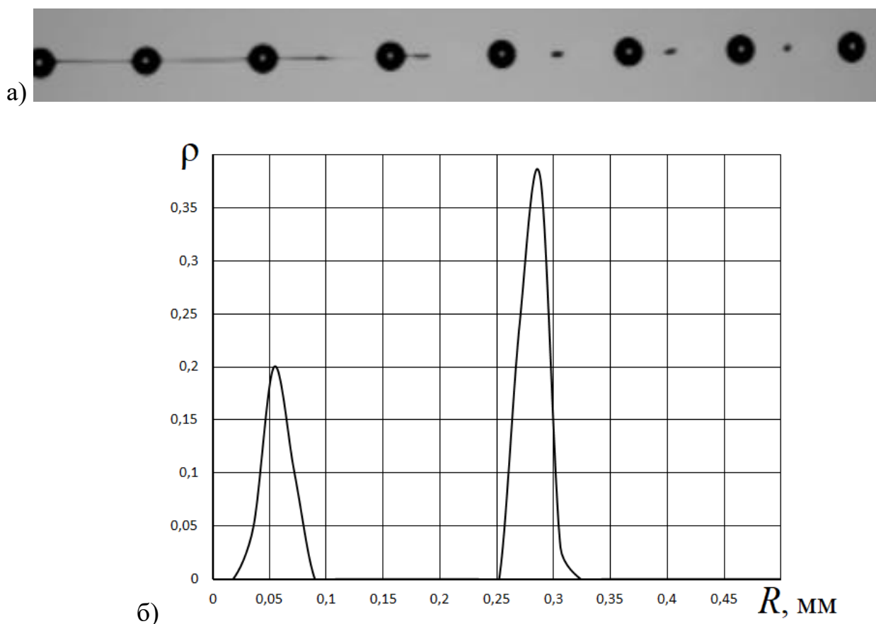
Рисунок 2.13. Параметры ВКРС: r_0 = 0,115 мм, On = 0,61 , k = 0,39 ; а) фотография распадающейся струи; б) функция распределения капель по размерам \Psi(R) .
