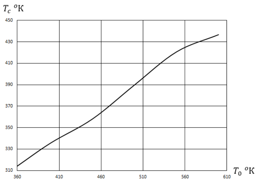
Рисунок 3.26. Зависимость конечной температуры оптимальной структуры от начальной температуры капельного потока; радиус капель в потоке – 100 мкм.
