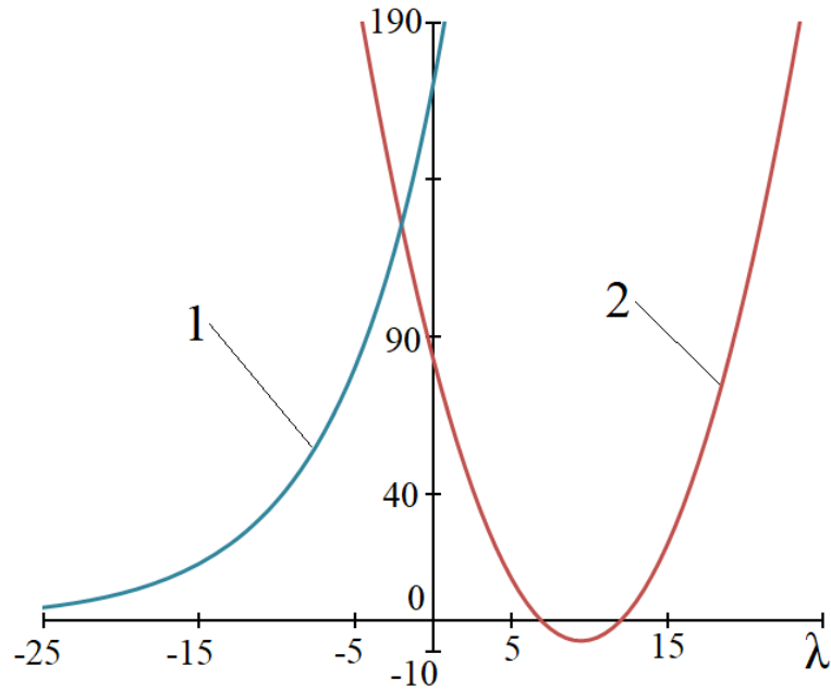
Рисунок 4.7. Решение системы уравнений (4.27) для \psi_1=0,3 , \psi_2=0,12 , \varphi_1=0,85 , \varphi_2=0,3 , w=0,3 : 1 – зависимость (\lambda^2 - a\lambda + b) ; 2 – зависимость d(1+4w)^2 e^{\lambda w/2} .
