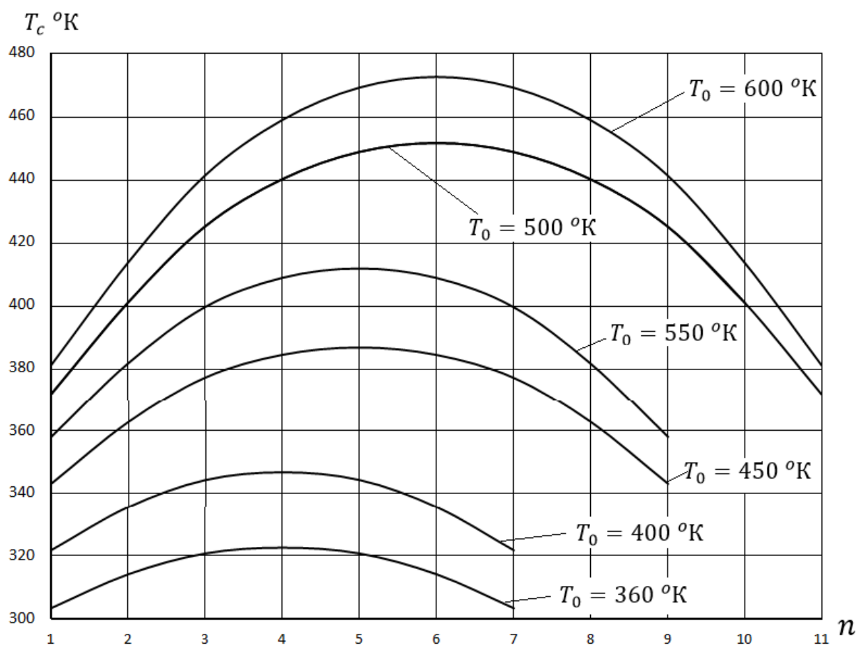
Рисунок 3.36. Распределение конечной температуры капель КХИ по толщине капельного потока для разных начальных температур. По оси абсцисс отложен номер капельной плоскости, по оси ординат – температура капель. Рабочее тело – вакуумное масло ВМ1, упаковка капель квадратная (расстояние между каплями – 4,76 r ), длина пролёта – 22 м.
