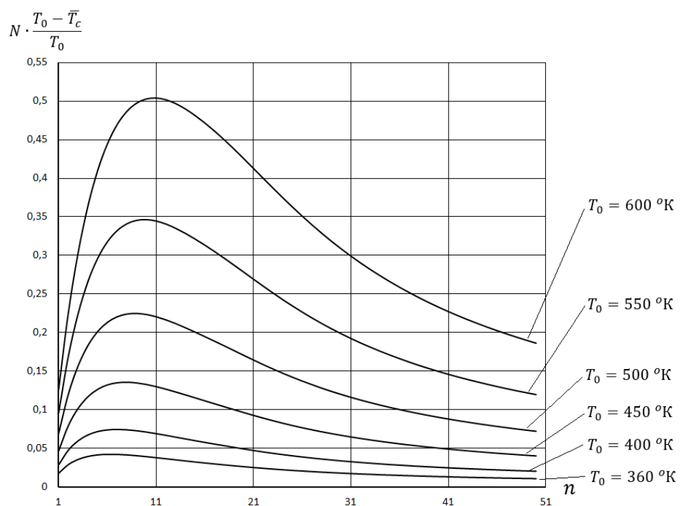
Рисунок 3.24. Зависимость \Pi = N \frac{T_0 - \bar{T}_c}{T_0} в МВТ от количества капельных плоскостей для разных начальных температур.
