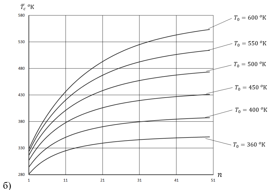
Рисунок 3.24. а) Зависимость тепловой мощности КХИ от количества капельных плоскостей в потоке, рассчитанная для разных начальных температур капель. б) Зависимость конечной среднемассовой температуры капель \bar{T}_k от количества капельных плоскостей для разных начальных температур.
