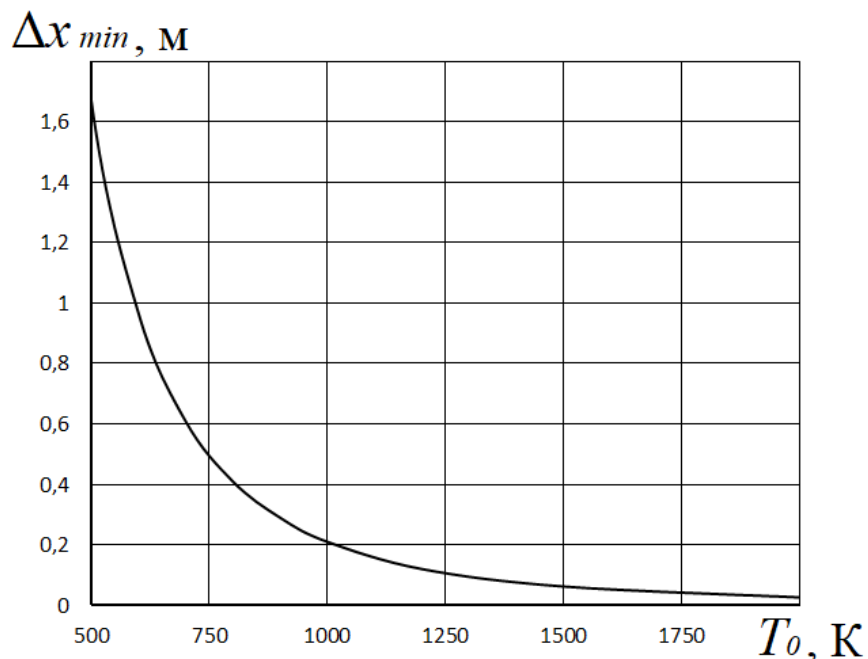
Рисунок 4.8. Зависимость \Delta x_{\min}(T_0) . \psi_1=0,3 , \psi_2=0,12 , \phi_1=0,85 , \phi_2=0,3 , r = 100 мкм, \rho = 800 кг/м 3 , c = 800 Дж·кг/К, u = 2 м/с.
