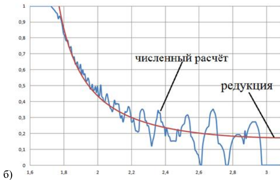
Рисунок 3.13. а) Схема редукции. б) Индикатрисы излучения для капельной плоскости, одна из которых получена численно, а другая рассчитана с использованием предложенного метода.
