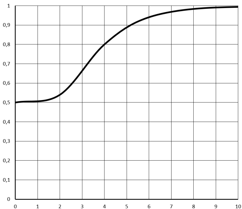
Рисунок 3.9. Зависимость коэффициента излучения капли и полубесконечной капельной плоскости от расстояния до края полуплоскости, \beta=\gamma=4,76 . Расстояние на графике отложено в единицах h .
