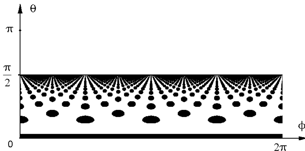
Рисунок 3.10. Результат расчета f при \beta=\gamma=4,76 , h = 20 . В закрашенных областях f=1 , в не закрашенных f=0 .
