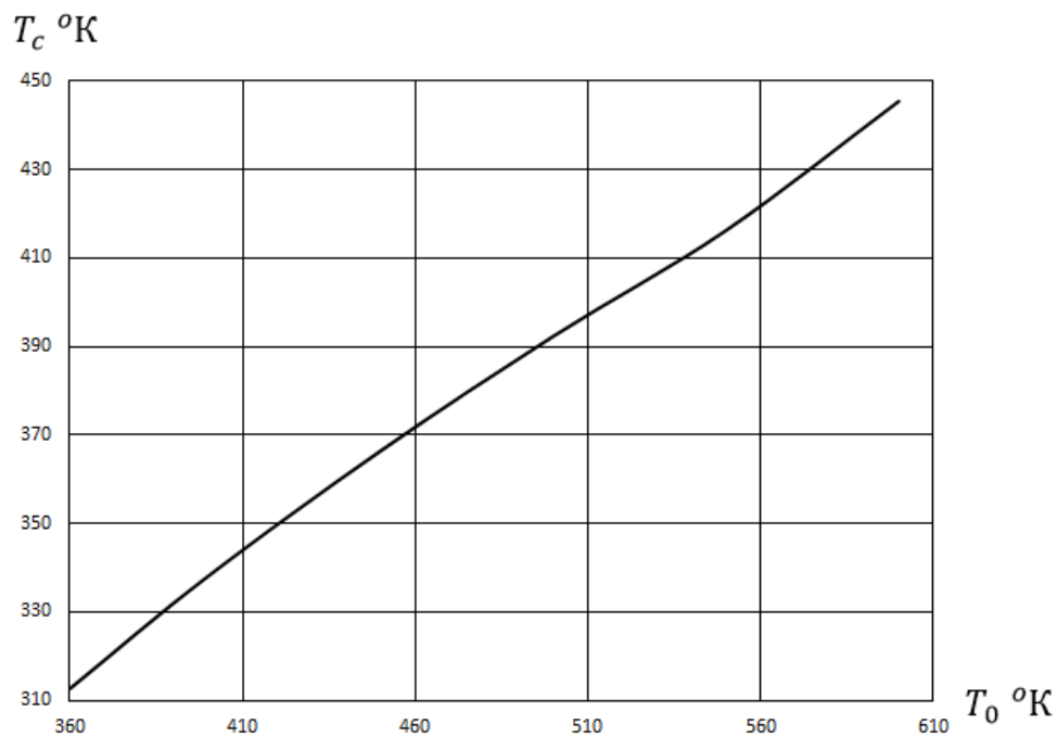
Рисунок 3.29. Зависимость конечной температуры оптимальной структуры от начальной температуры капельного потока.
