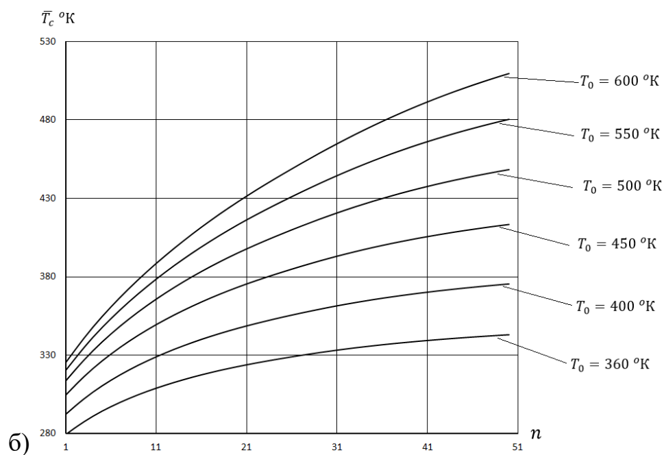
Рисунок 3.27. а) Зависимость тепловой мощности КХИ от количества капельных плоскостей в потоке, рассчитанная для разных начальных температур капель. б) Зависимость конечной среднемассовой температуры капель \bar{T}_K от количества капельных плоскостей для разных начальных температур.
