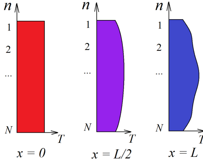
Рисунок 4.2. Процесс установления профиля температуры капельного потока.
