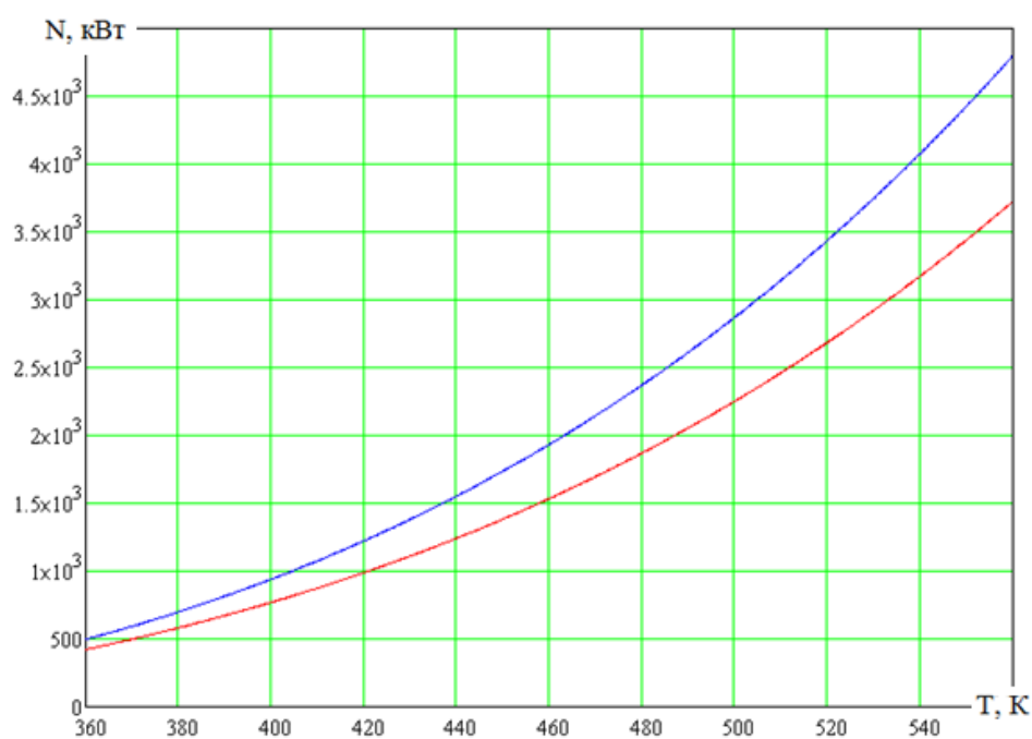
Рисунок 3.23. Зависимость тепловой мощности КХИ от T_0 при перепаде температуры рабочего тела 50К: — с учётом переоблучения элементов конфигурации, — без учёта переоблучения элементов конфигурации.
