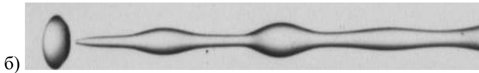
Рисунок 2.6. Характерный автомодельный профиль струи при малых Oh < 0,2 : а) аналитически рассчитанная зависимость; б) фотография эксперимента с водой.
