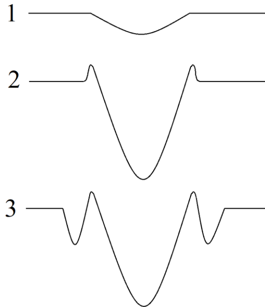
Рисунок 2.25. Стадии формирования фрактального профиля струи.
