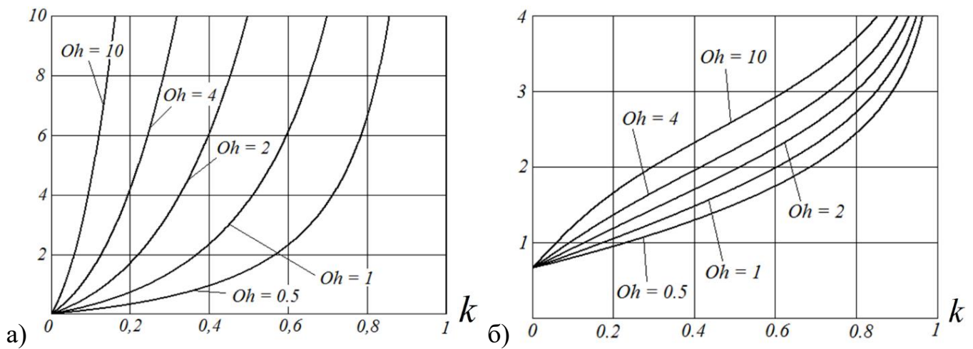
Рисунок 7. а) Зависимость отношения вязкого члена уравнения (2.54) к инерционному от k для разных Oh при f = 0,4 . б) Зависимость десятичного логарифма отношения сил поверхностного натяжения уравнения (2.52) к инерционному от k для разных Oh при f = 0,4 .
