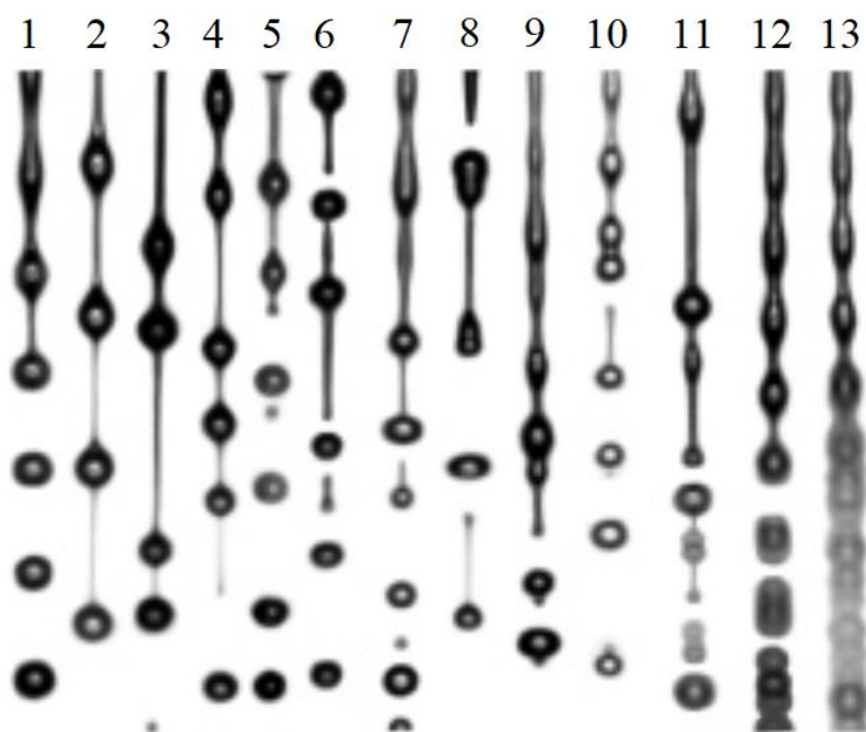
Рисунок 1.11. Поведение струи вблизи точки распада [80].
