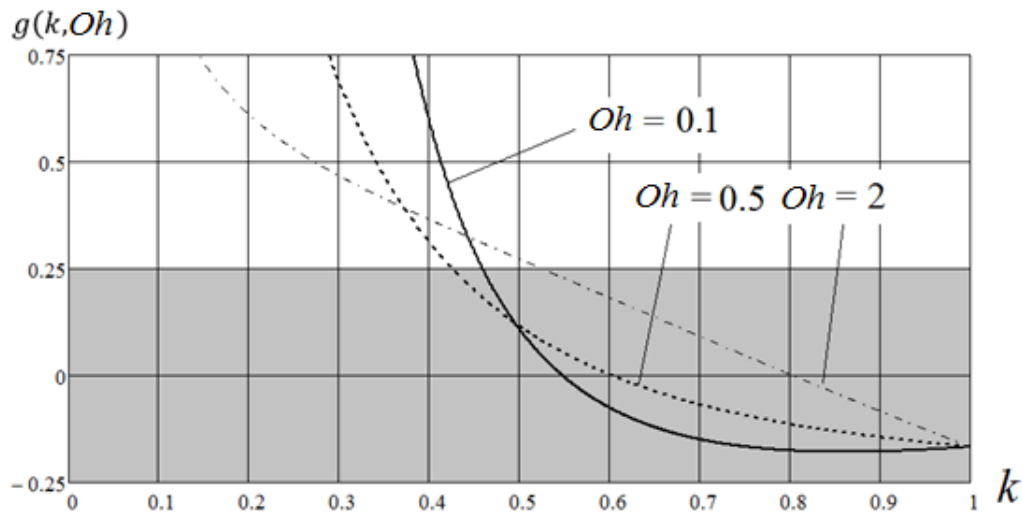
Рисунок 2.3. Зависимость g(k) , рассчитанная для разных значений Oh . Закрашенная область соответствует безсателлитному распаду.
