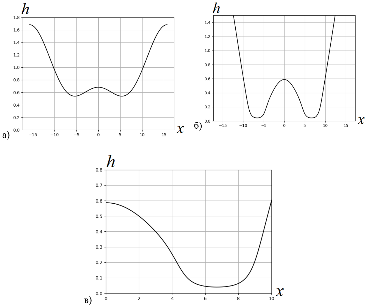
Рисунок 2.18. Зависимость формы струи от координаты в различные моменты времени: а) t = t^* - 3,94 ; б) и в) t = t^* - 1,05 .
