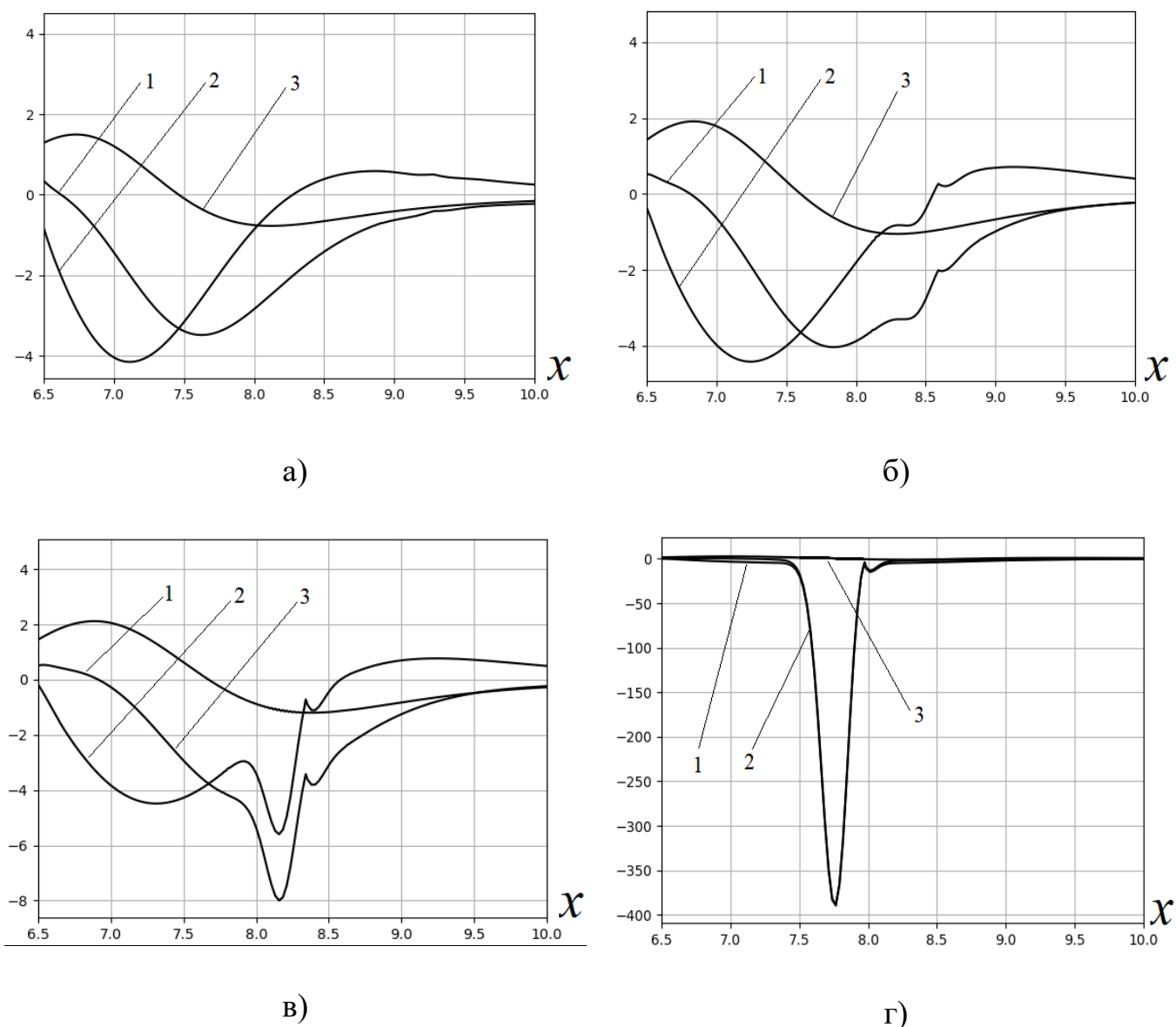
Рисунок 2.22. Соотношение функций (\eta_1 + \eta_2) , \eta_2 и \eta_3 для различных моментов времени: 1– (\eta_1 + \eta_2) ; 2– \eta_2 ; 3– \eta_3 . а) \Delta t = 0,135 ; б) \Delta t = 0,081 ; в) \Delta t = 0,054 ; г) \Delta t = 0 .
