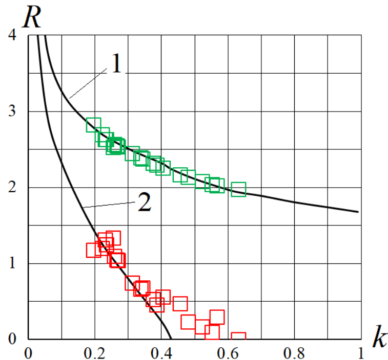
Рисунок 2.14. Линиями обозначена теоретически рассчитанная зависимость безразмерного радиуса 1 - основных и 2 - сателлитных капель от безразмерного волнового числа для случая On = 0,6 . Зелеными и красными квадратами – экспериментально измеренная зависимость радиуса капель от безразмерного волнового числа при On = 0,6 \pm 0,15 .
