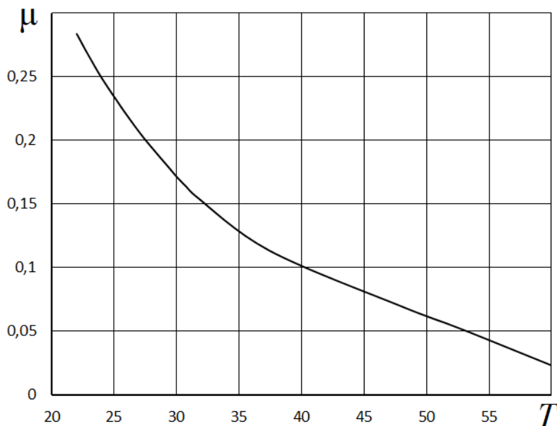
Рисунок 2.12. Зависимость динамической вязкости вакуумного масла ВМ1-С от температуры T (выражена в градусах Цельсия).
