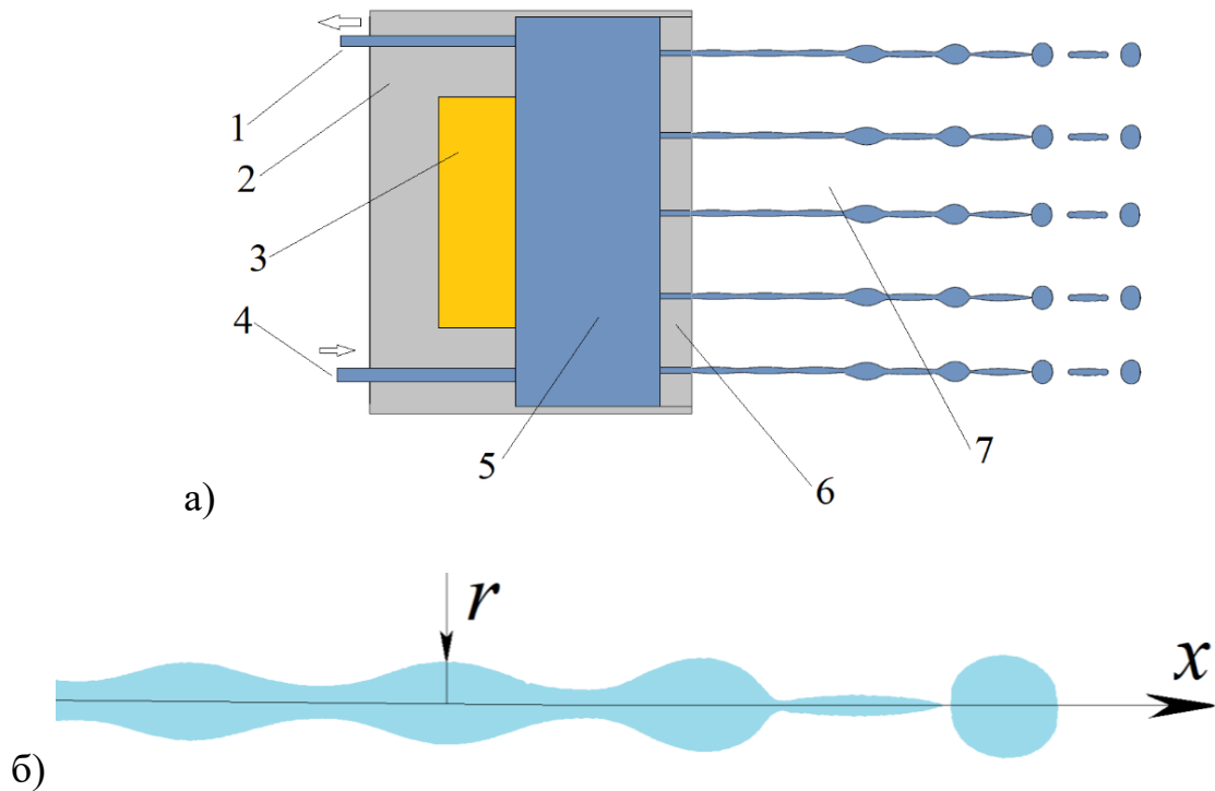
Рисунок 2.1. а) Принципиальная схема генератора капель. 1, 4 – подводящие и отводящие рабочее тело трубопроводы; 2 – корпус; 3 – пьезоэлемент; 5 – внутренняя камера; 6 – фильера с капиллярными отверстиями; 7 – распадающиеся на капли струи. б) Процесс капиллярного распада струи.
