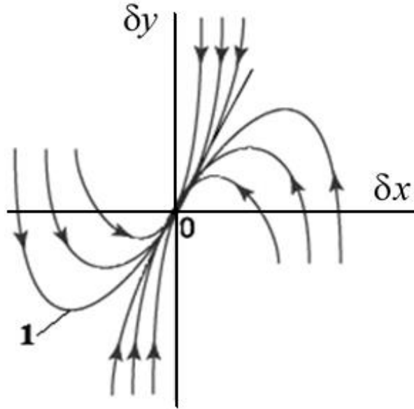
Рисунок 4.4. Решения системы (12) вблизи особой точки. Цифрой 1 обозначена траектория системы с немонотонным изменением безразмерной температуры.
