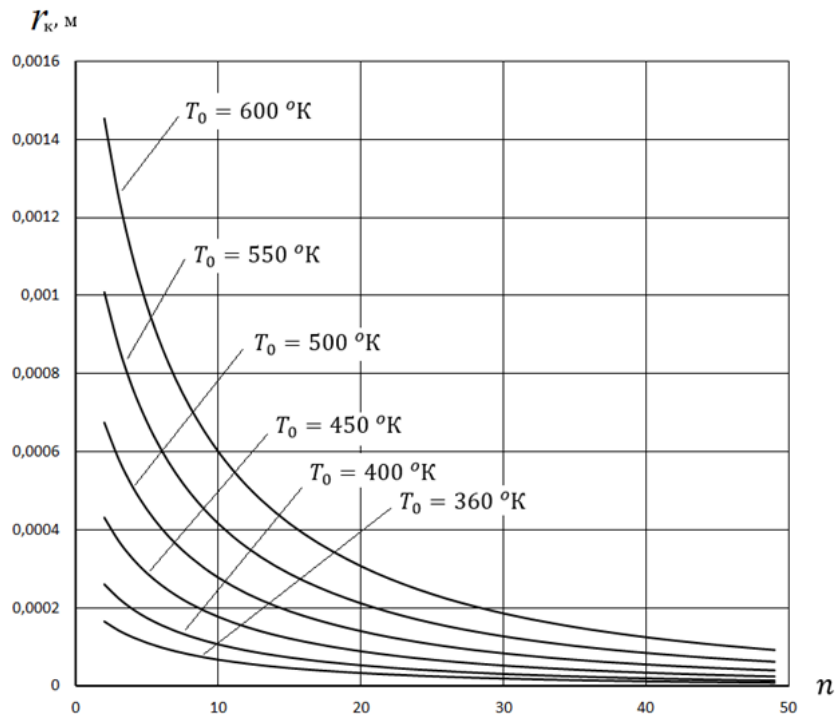
Рисунок 3.32. Зависимость радиуса капель КХИ от количества капельных плоскостей в капельном потоке для разных начальных температур. Разница между начальной температурой и конечной среднемассовой составляет 50 К.
