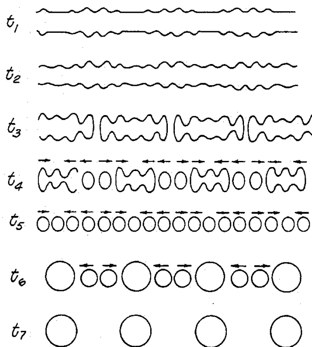
Рисунок 1.6. Схема образования монодисперсного капельного потока при двухмодовом распаде.
