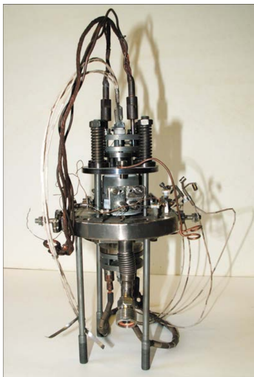
Рис. 1. ТЭП с плоской геометрией электродов для измерения ВАХ в смеси паров цезия и бария и изучения его работы с промежуточным электродом между эмиттером и коллектором в режиме полностью управляемого вентиля для преобразования постоянного тока реактора-генератора в переменный ток.
