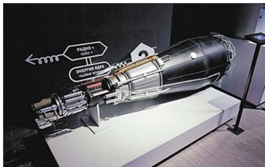
Рис. 5. Общий вид установки "Топаз" в демонстрационном зале политехнического музея.
